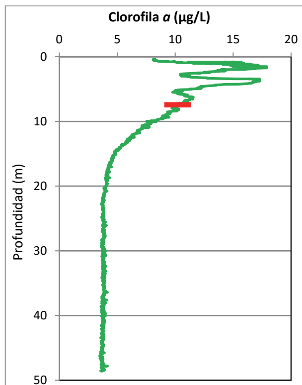
Figura 6. Perfil vertical de la clorofila a. Nótese las diferentes escalas para el muestreo de junio (a la izquierda) y septiembre (a la derecha).
