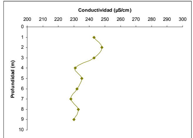
GRÁFICO 1 PERFILES FÍSICO-QUÍMICOS DEL EMBALSE DE TERRADETS
