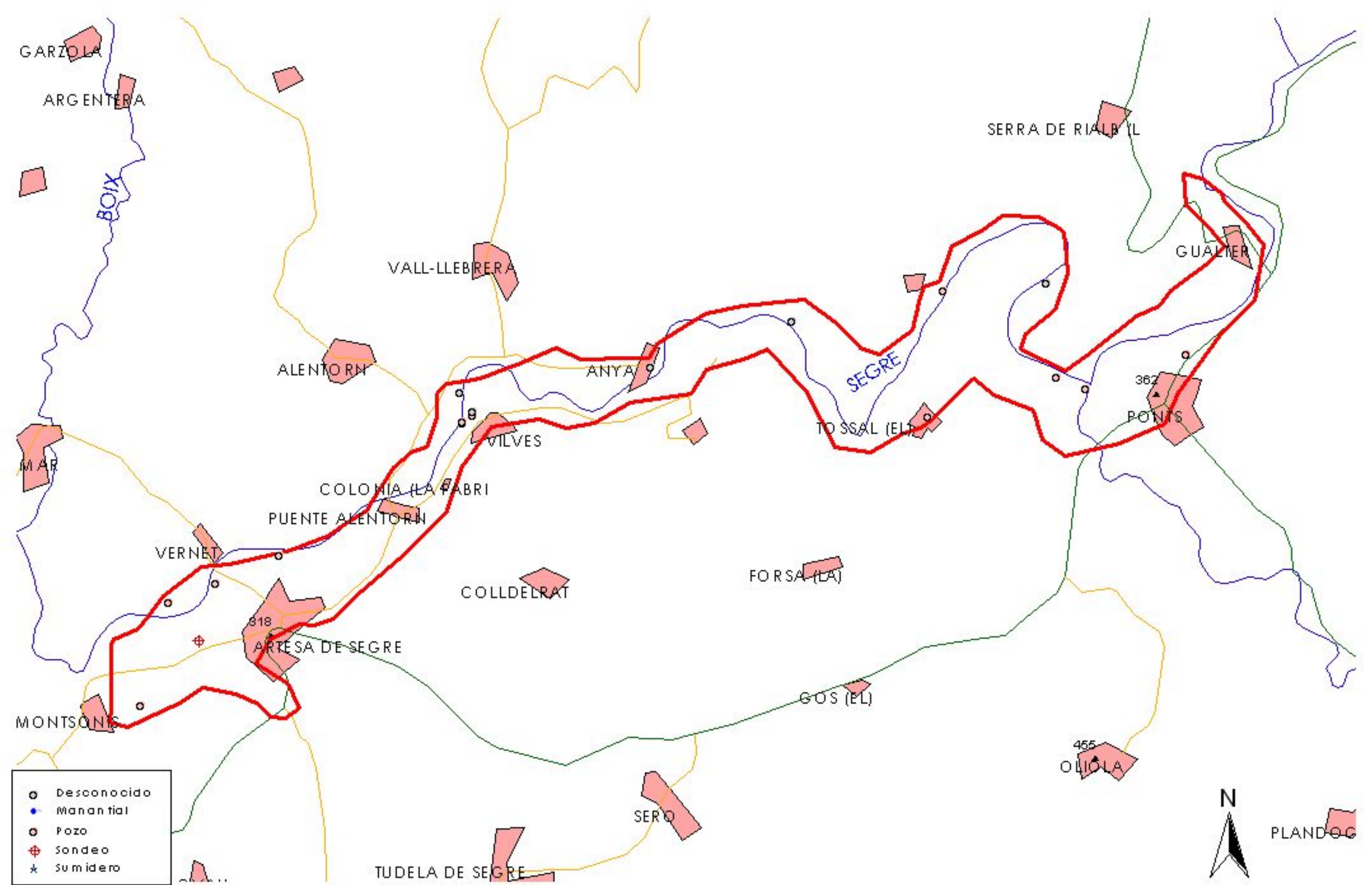
MAPA 9.2: MAPA DE INVENTARIO DE PUNTOS DE AGUA 90_062 ALUVIAL MEDIO SEGRE
