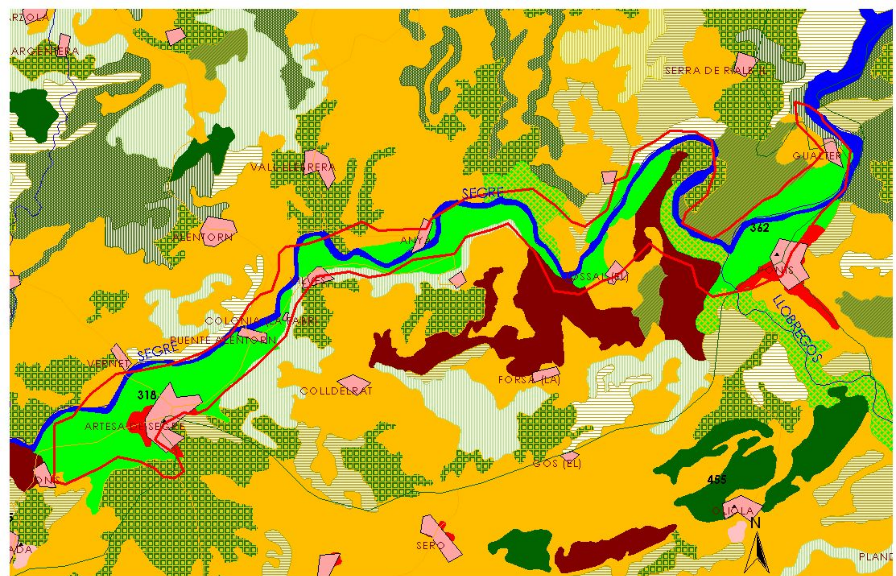
MAPA 13: MAPA DE USOS DEL SUELO 090_062 ALUVIAL DEL MEDIO SEGRE
