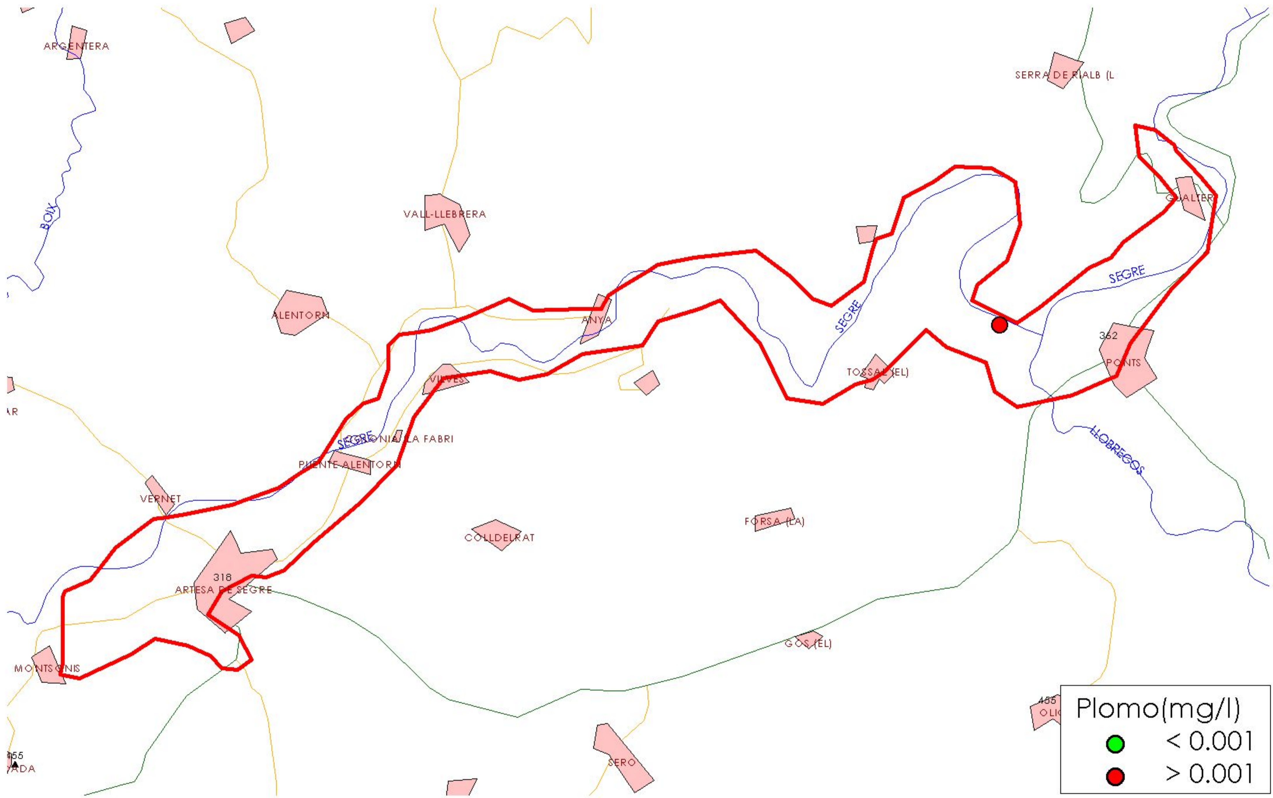
MAPA 10.5.2: MAPA DE NIVELES DE REFERENCIA 90_062 ALUVIAL DEL MEDIO SEGRE
