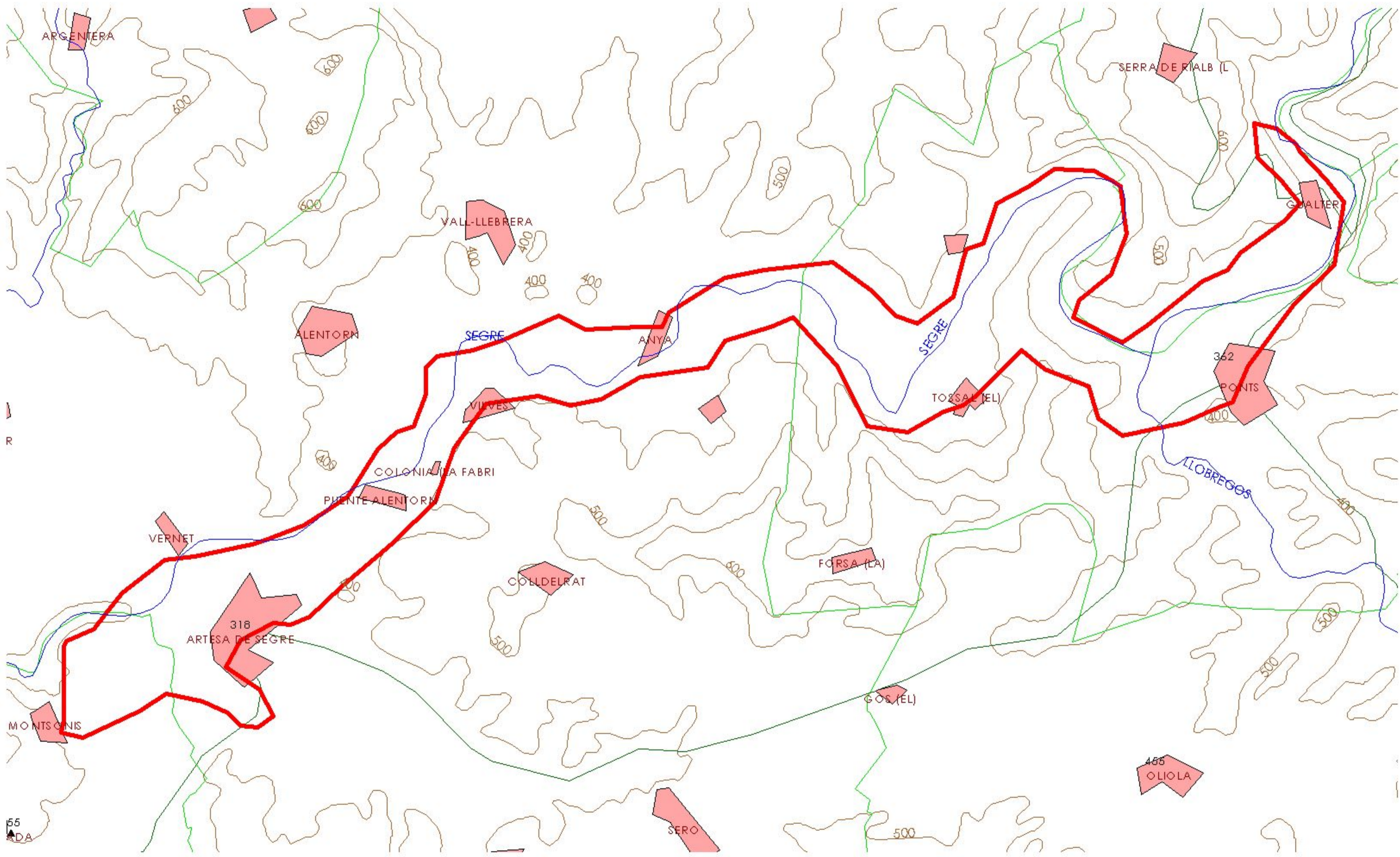
MAPA 1.1: MAPA DE IDENTIFICACIÓN 90_062 ALUVIAL DEL MEDIO SEGRE
